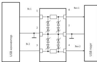
Типовая схема применения модуля МКМ055 для защиты двух линий высокоскоростного интерфейса
