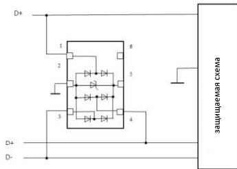
Схема применения модуля МКМ035 для защиты одной дифференциальной и одной несимметричной высокоскоростной линии связи
