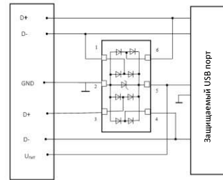
Рекомендуемая схема защиты порта USB с помощью модуля типа МКМ025
