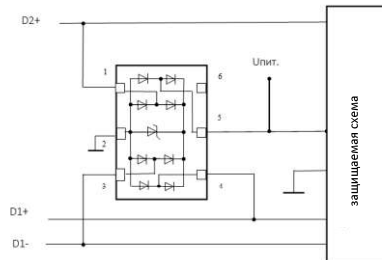
Схема применения модуля МКМ045 для защиты одного дифференциального и одного несимметричного высокоскоростного канала связи, а также источника питания
