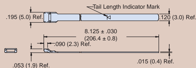
Micro-Band 600-057 Precoiled Micro-Band 600-057-1
