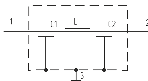
Рис.2 Схема Pi-фильтра
